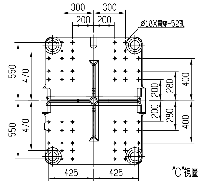
前模板與押出關係圖說明
