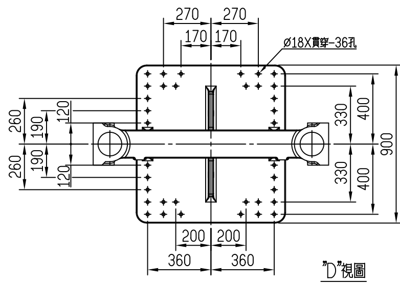
中模板與押出關係圖說明
